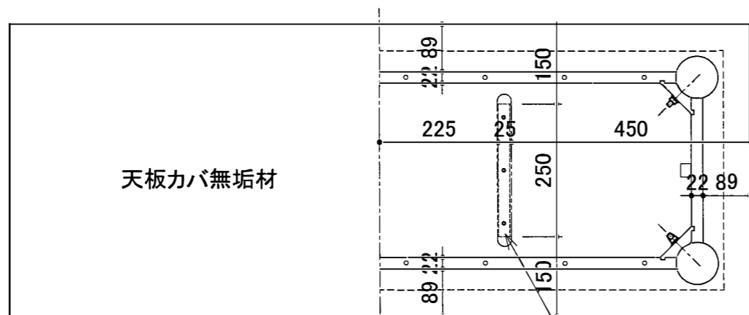
反り止めLアンクル (250×25×15×2.3)2本
