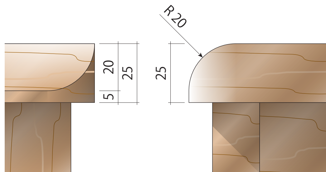
天板 詳細図 Scale = 1 : 2
