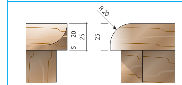
天板 詳細図 Scale = 1 : 2
